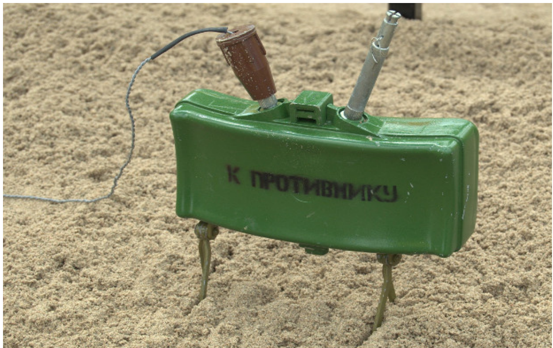
Мина в боевом положении
